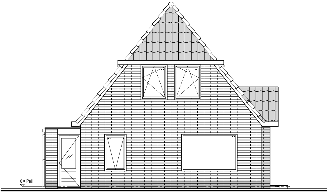
Linker zijgevel
