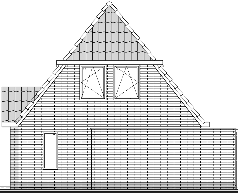
Rechter zijgevel
